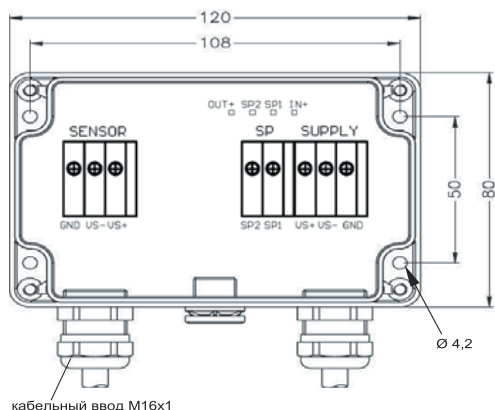
Пластмассовый корпус
