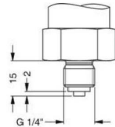
Код 400 (G1/4" EN 837-1/-3)
